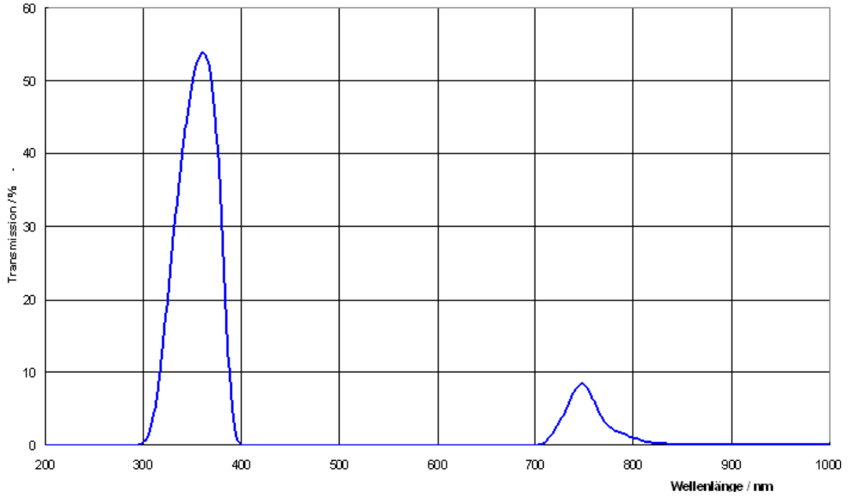
UG 1, Dicke 3 mm
