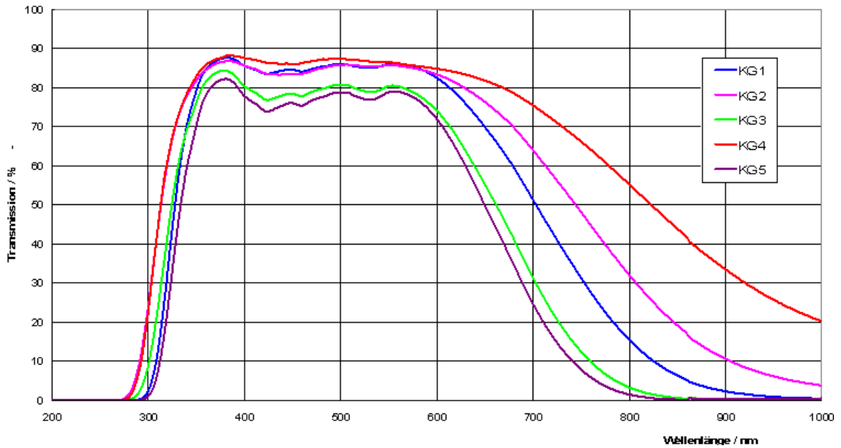
KG-Filter, IR-Bereich, Dicke 3 mm
